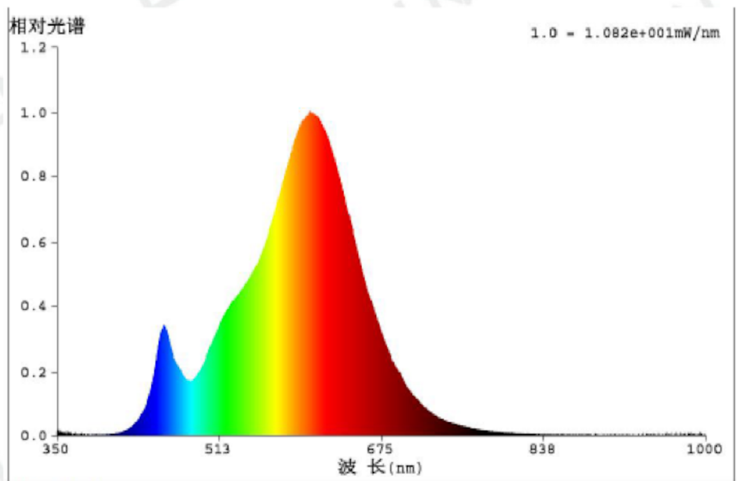
光谱分布
